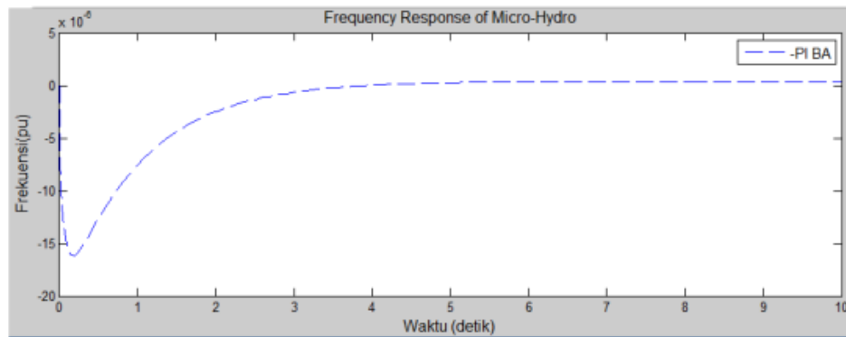
Gambar 4. Simulasi pembangkit mikrohidro dengan PI-BA
