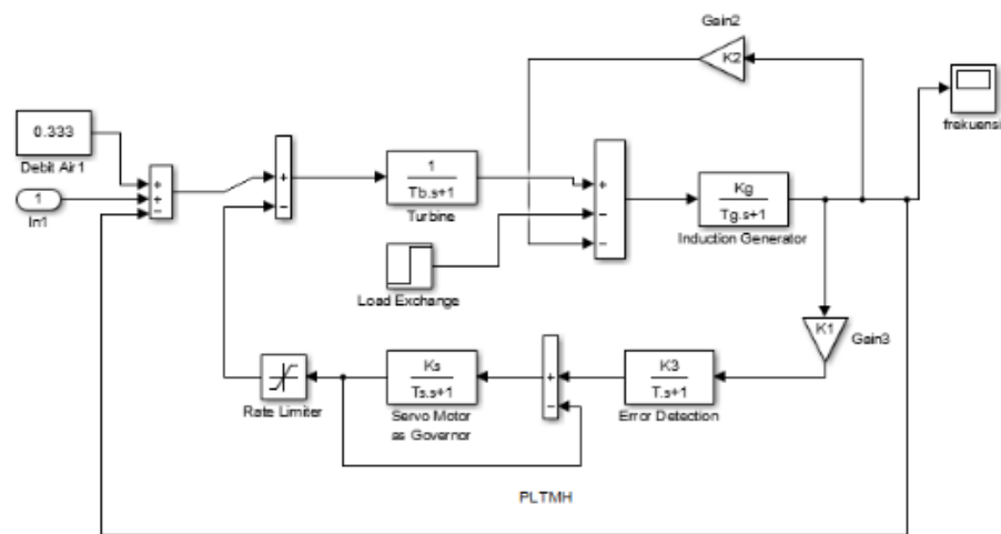
Gambar 1. Pemodelan pembangkit mikrohidro
